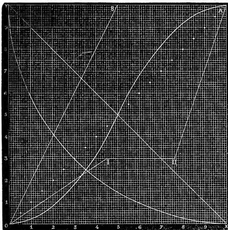
Fig. 121. — Expressions graphiques de mouvements de différentes natures. — OX' axe des X ou des abscisses ; 1, 2, 3, 4, etc., divisions du temps en secondes. — OY axe des Y ou ordonnées ; 1, 2, 3, 4, etc., divisions de l'espace en mètres. — Ligne ponctuée AO , mouvement uniforme lent ascendant. — OB , mouvement uniforme ascendant plus rapide. — OIII , combinaison de mouvements ascendants et d'arrêt ; OI , mouvement uniforme lent ; III , arrêt ; HA , mouvement uniforme rapide. — OA , ligne courbe : mouvement ascendant accéléré puis diminué. — YX (ligne droite), mouvement uniforme descendant. — YX (ligne courbe), mouvement descendant diminué.
